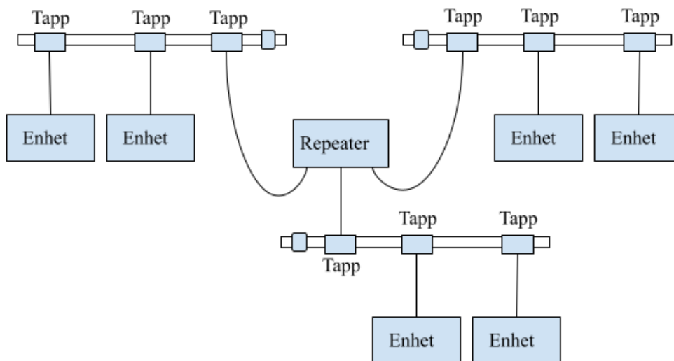
Figur 2.11: ControlNet stjärntopologi
